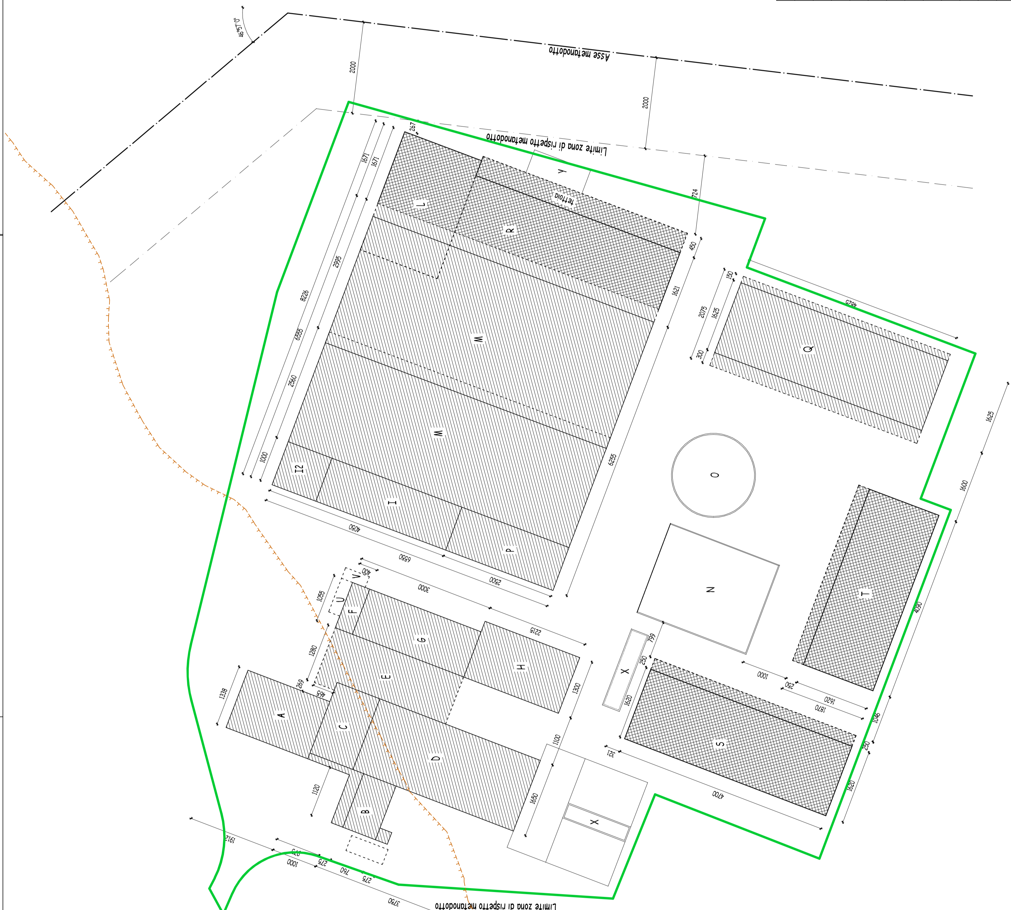
Pianimetria aziendale di fatto scala 1:500
