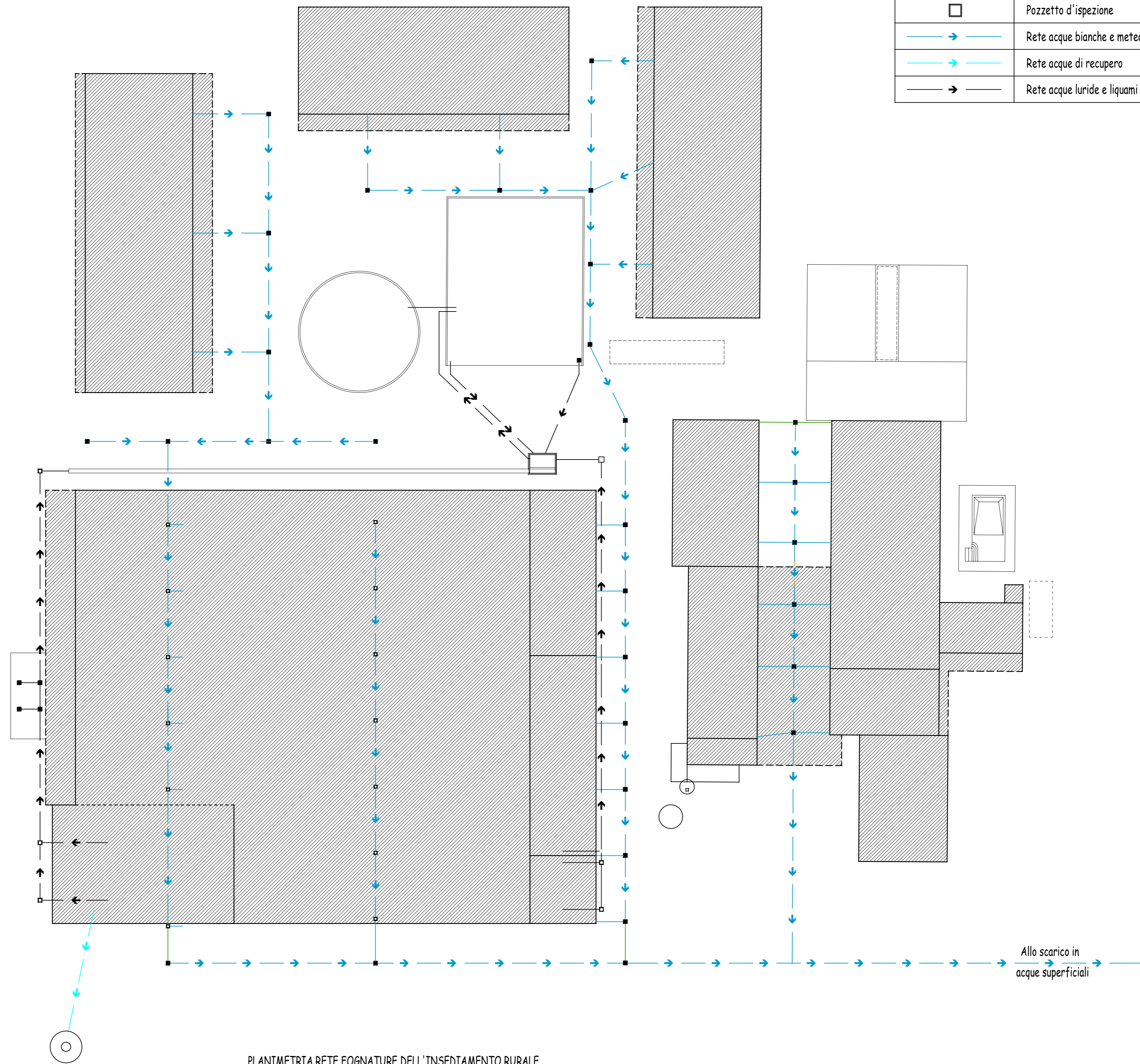
PLANIMETRIA RETE FOGNATURE DELL'INSEDIAMENTO RURALE
