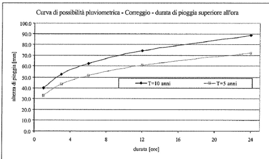
Figura 2: curve di possibilità pluviometrica per il Comune di Correggio per durate di pioggia superiori all'ora
