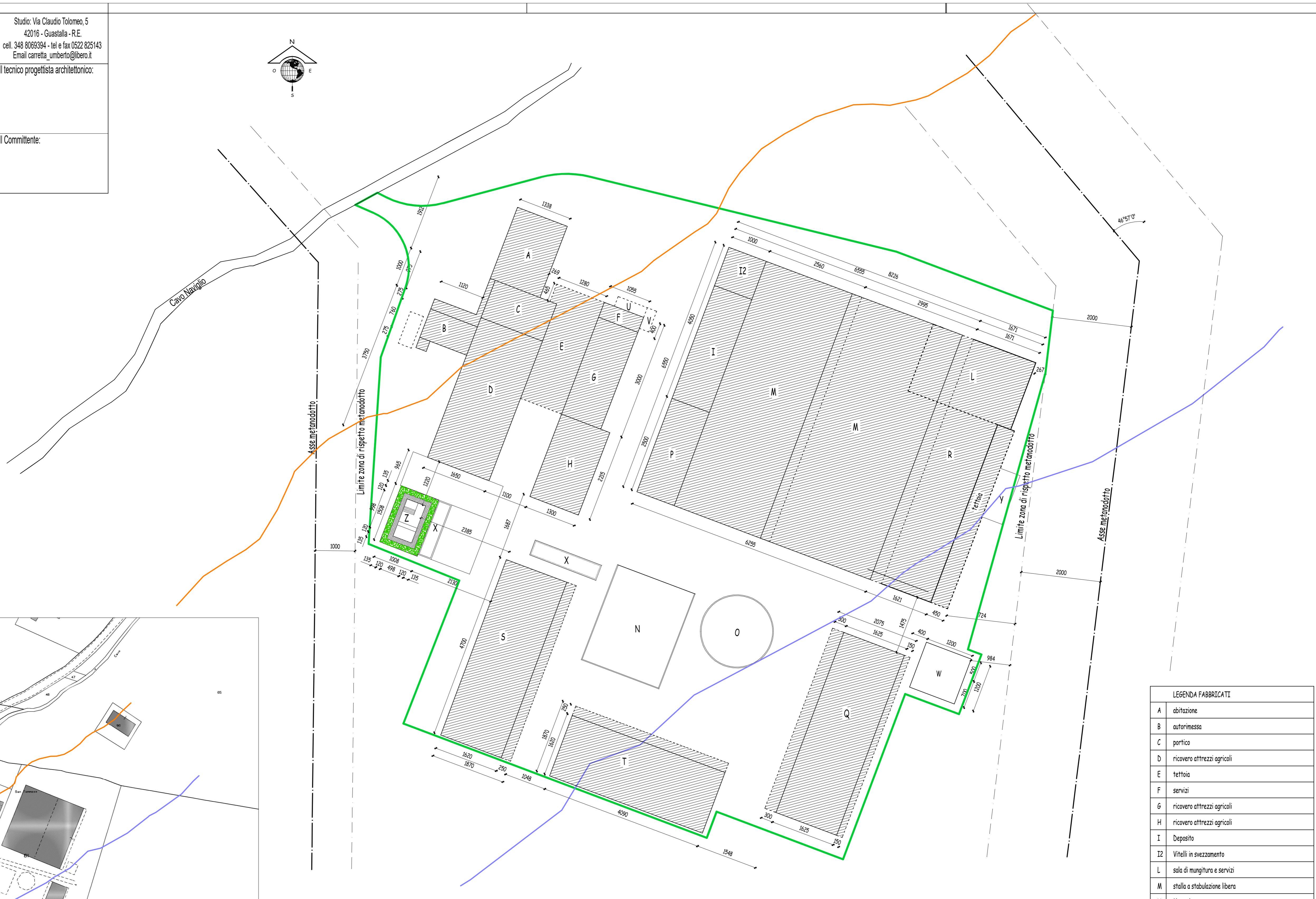
Planimetria aziendale di fatto scala 1:500
