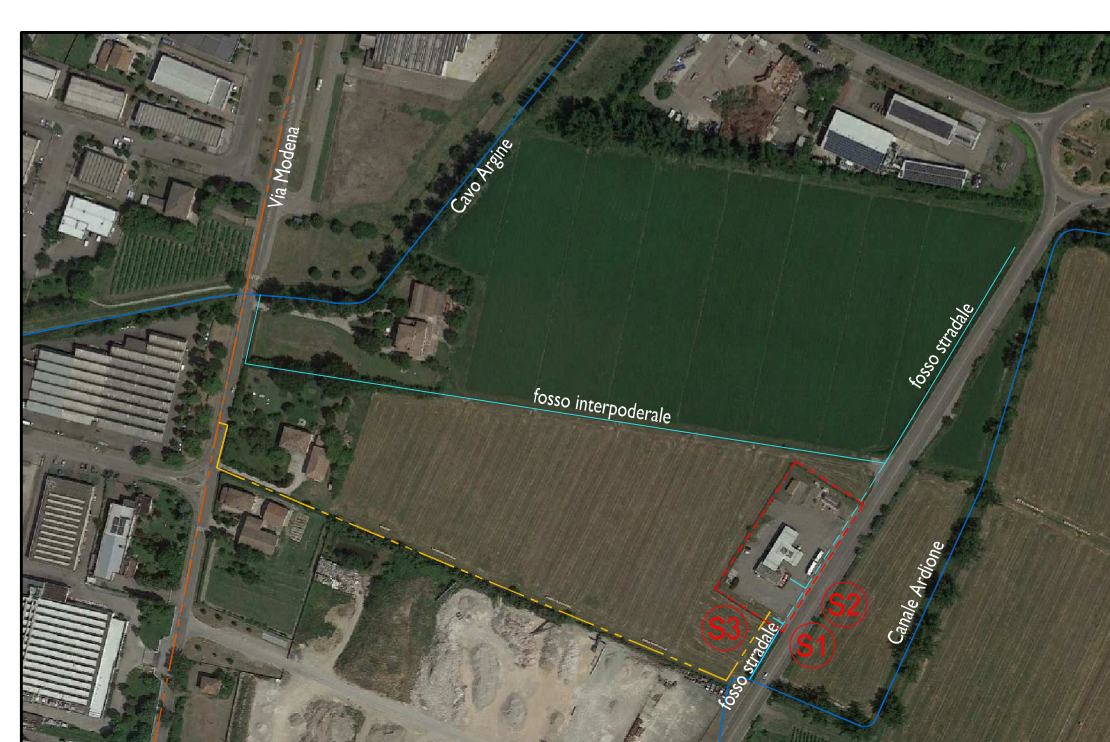
STATO DI FATTO: RETE FOGNARIA (SCALA 1:5.000)
