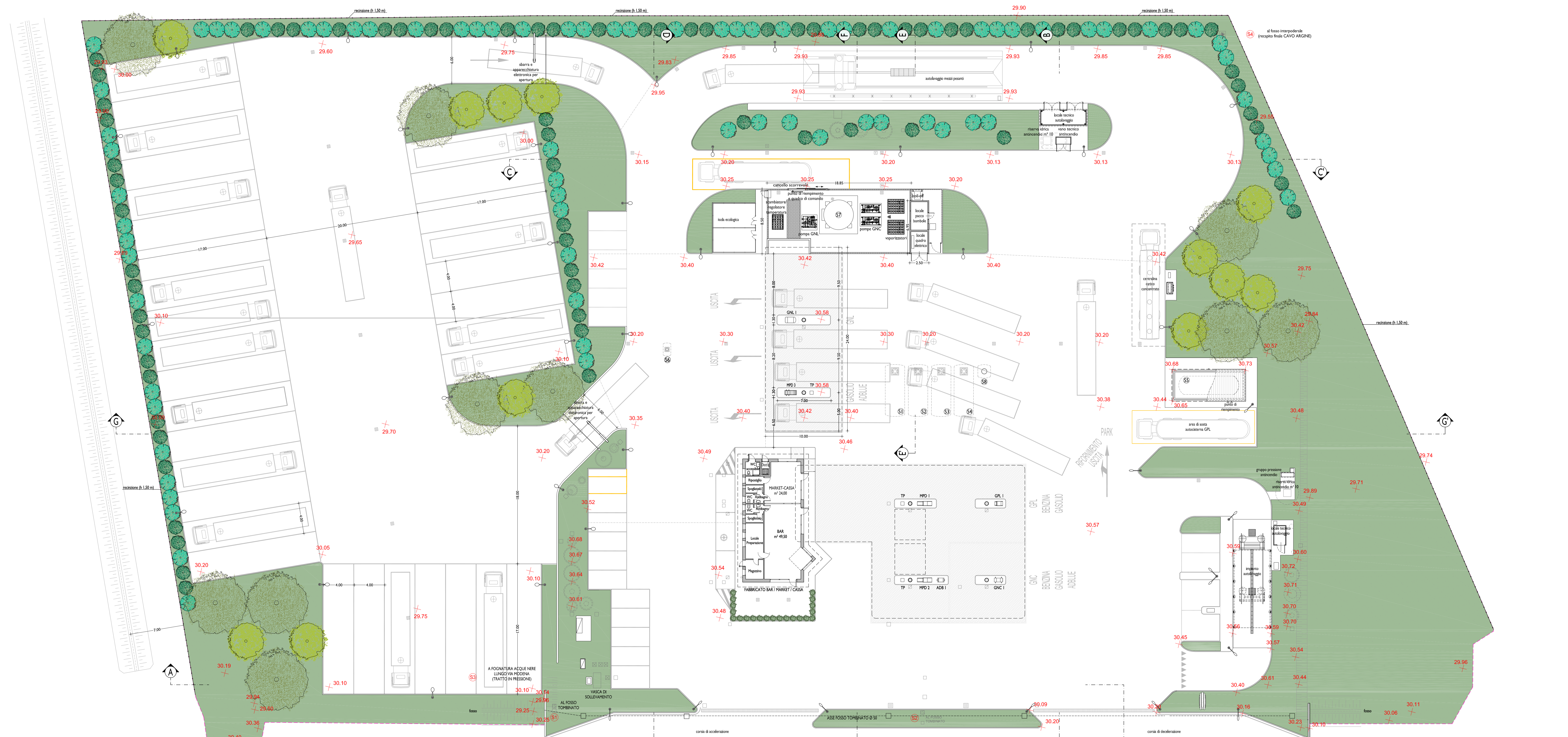
PROGETTO: PLANIMETRIA GENERALE (SCALA 1:200)
