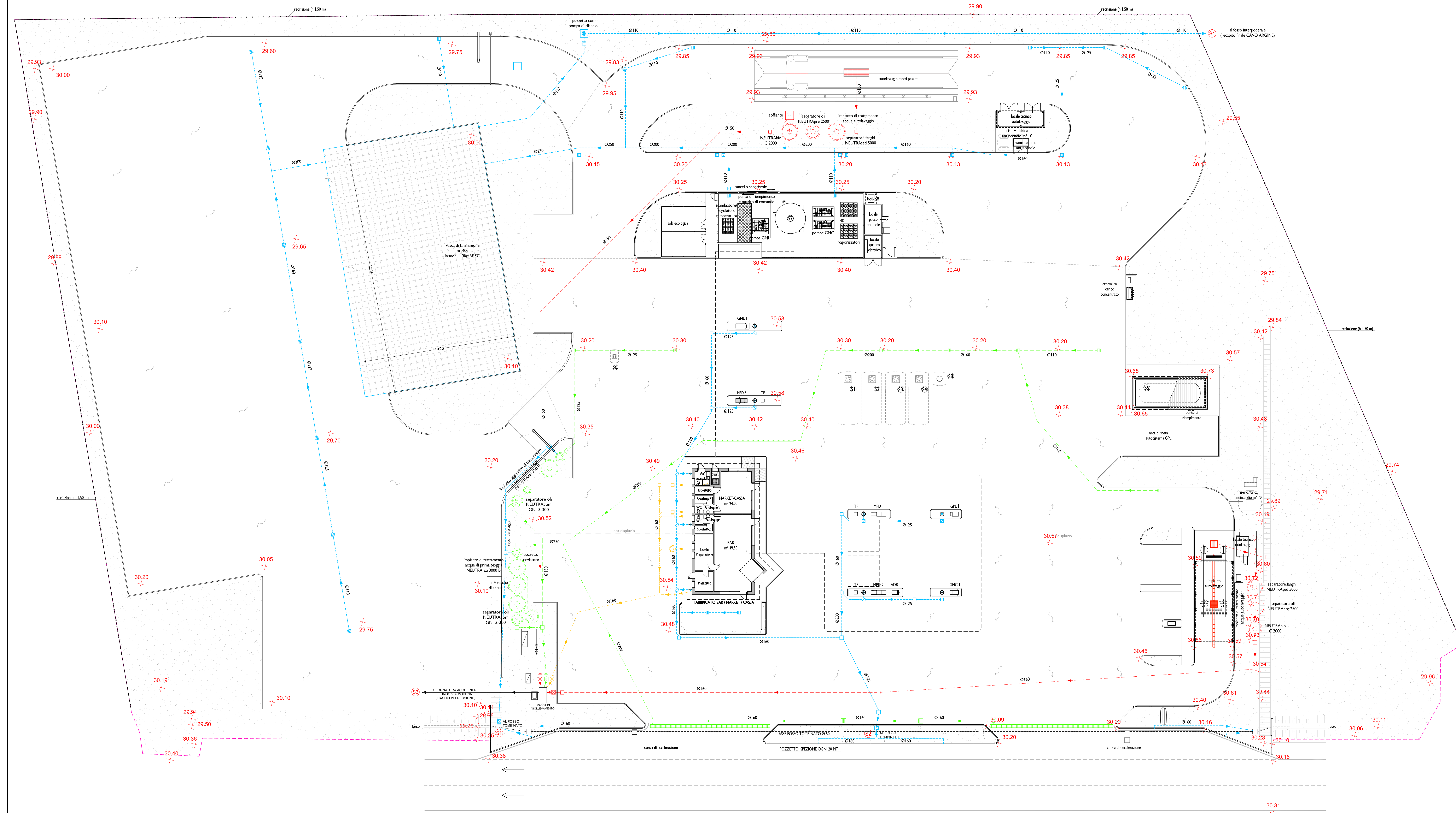
PROGETTO: PLANIMETRIA GENERALE IMPIANTO FOGNARIO (SCALA 1:200)
