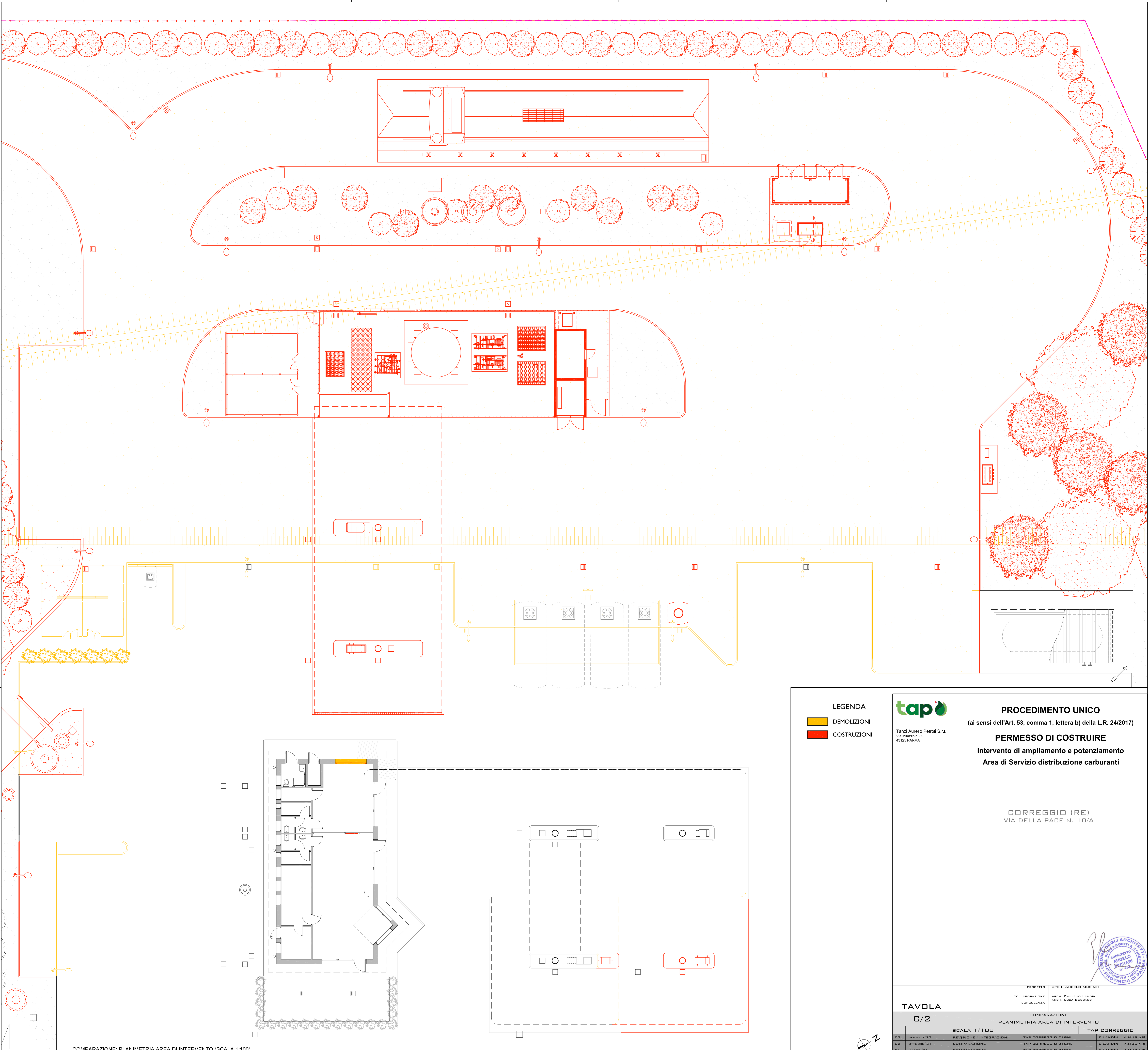
COMPARAZIONE: PLANIMETRIA AREA DI INTERVENTO (SCALA 1:100)
